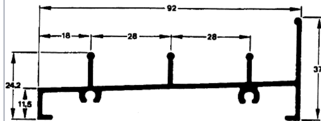
MP-367 0.818 Kg/m Marco Inferior
