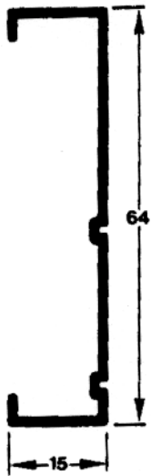
MP-359 0.363 Kg/m Marco Lateral para Bandeira
