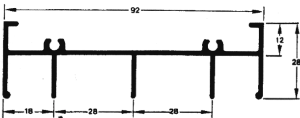
MP-366 0,865 Kg/m Marco Superior
