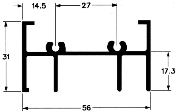
MP-342 0,655 Kg/m
