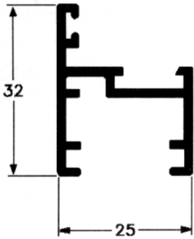
MM-375/25304 0,417 Kg/m
