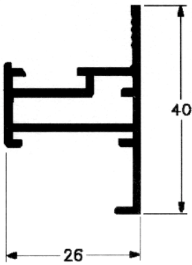
MM-375/25304 0,417 Kg/m
