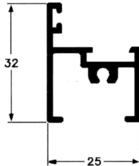
25-315 0,434 Kg/m
