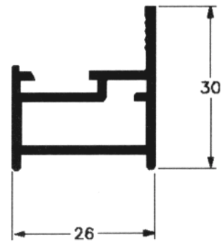
25-314 0,363 Kg/m
