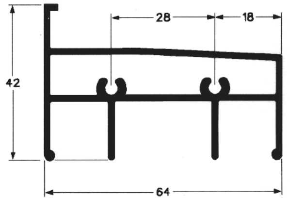
MP-388 0,905 Kg/m
