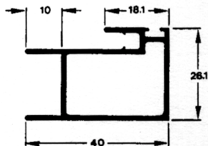
MP-303 0.474 Kg/m Montante com engate Veneziana
