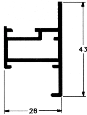
25-315 0,434 Kg/m
