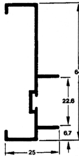
MP-360 0,442 Kg/m Marco Lateral/Porta e Janela
