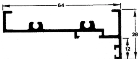
MP-363 0.539 Kg/m Marco
