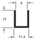
ALT-44 Perfil U 0,130 kg/ml
