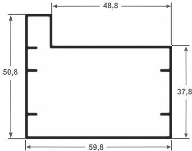
ALT-PC026 Portão 0,731 kg/ml
