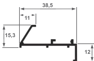
DS-005 (Z-063) 0,346 kg/ml
