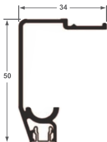
ALT-600 Trilho Superior 0,473 kg/ml
