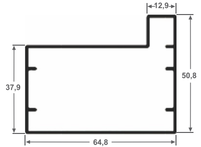
ALT-PC027 Portão 0,781 kg/ml
