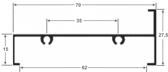
Z-175 Linha 25 0,533 kg/ml
