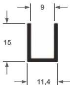
ALT-44 Trilho U 0,130 kg/ml
