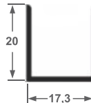
U-398 Uzinho 0,241 kg/ml
