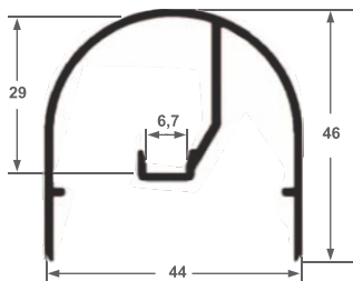
ALS-60 Chapéu 0,575 kg/ml
