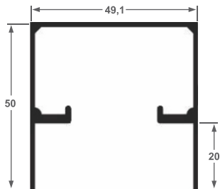
U-397 Chapéu 0,659 kg/ml
