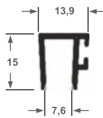
ALT-46 Vedação Transpasse 0,153 kg/ml
