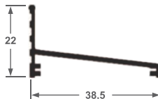
ALS-71 Trilho 0,264 kg/ml
