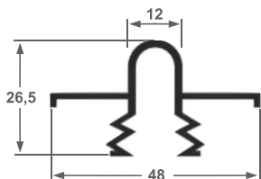
PC-006 (E-364) 0,501 kg/ml
