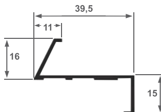
DS-006 (Z-033) 0,361 kg/ml
