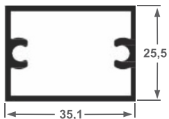
CG-012 (D-055) 0,598 kg/ml
