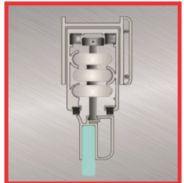
ALT-705 Leito vidro 10mm 0,525 kg/ml
