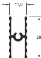
ALS-73 Travessa 0,234 kg/ml
