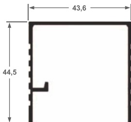
ALS-70 Chapéu 0,470 kg/ml
