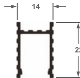
ALS-74 Montante 0,180 kg/ml
