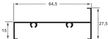
ALT-310 Portão 0,500 kg/ml
