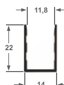
ALT-87 Perfil U Móvel 0,159 kg/ml
