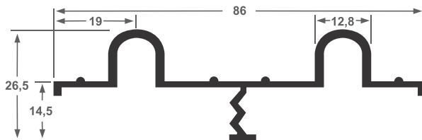
PC-005 (E-365) 0,656 kg/ml
